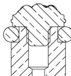
COUPE B-B
